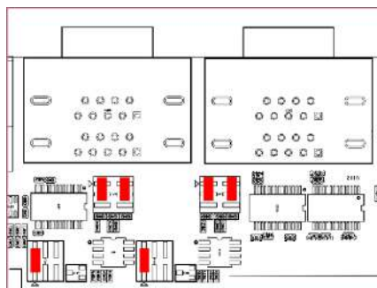
RS-232跳冒位置
