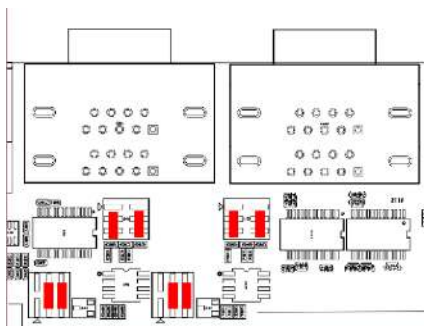
RS-485跳冒位置
